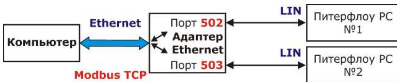
Рисунок 1: Адаптер Ethernet↔Прибор
