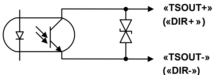
Рис.Б.1 - Схема окончного каскада универсальных выходов
