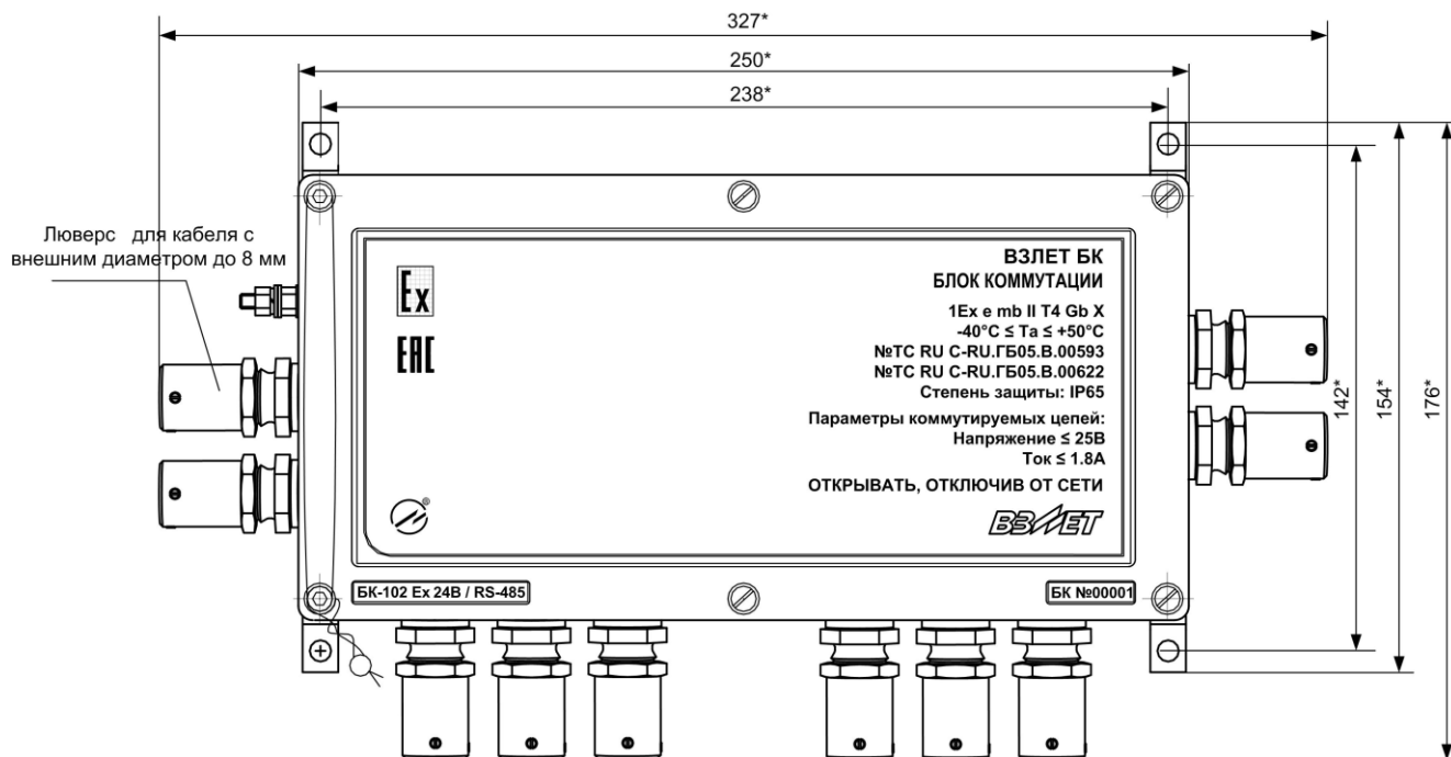
Рис.А.6 - Вид блока коммутации.
