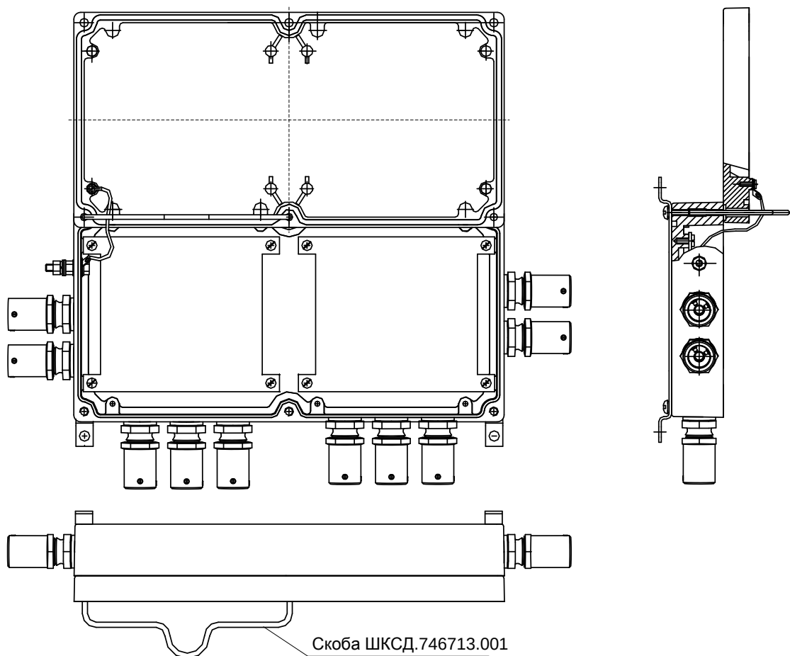
Рис.А.7 - Фиксация открытой крышки БК с помощью скобы.
