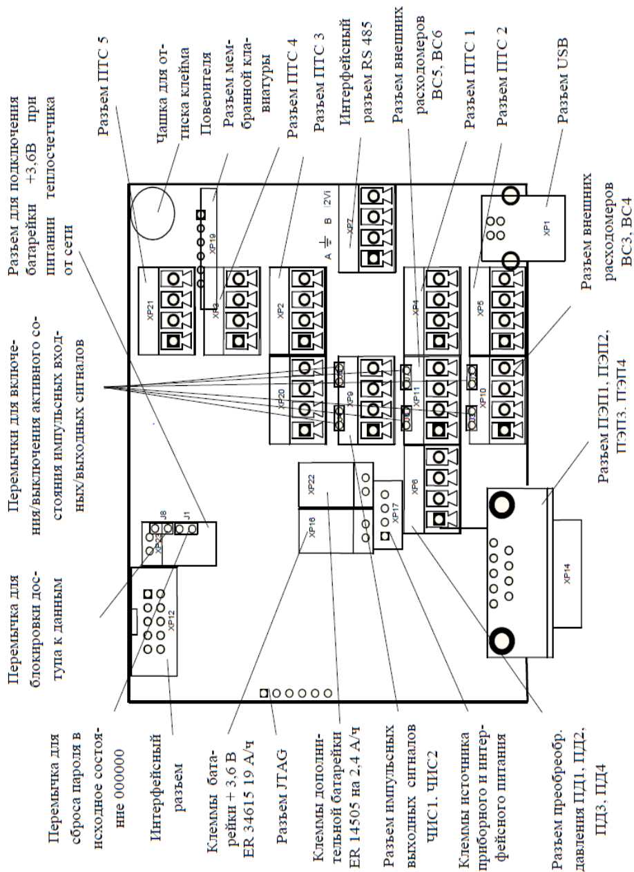
Рисунок 1 - Расположение разъемов и джамперов под крышкой СТУ-1 Модель ЭМ.1,3М.2
