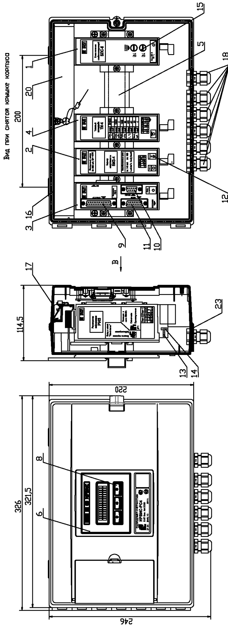
Габаритные и присоединительные размеры ВП ИРВИС-РС4М-Ультра* (корпусное исполнение)
