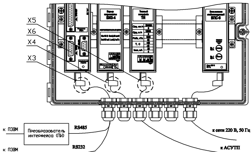
Верхняя крышка БИП снята
