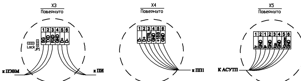
Рисунок 2 – Схемы подключения БИП расходомера-счетчика
