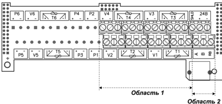
Рисунок Б.1 – Плата подключений вычислителя KAPAT-307-4V4TOP
