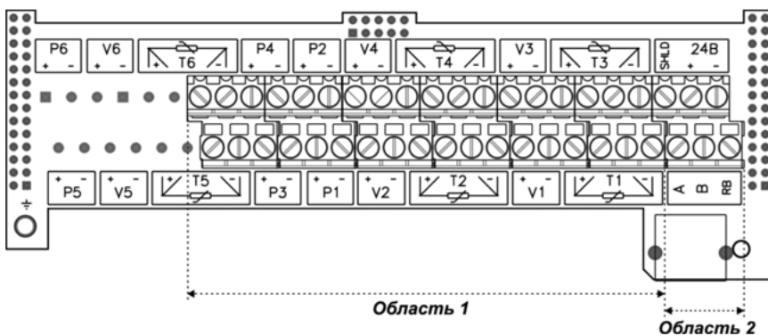
Рисунок Б.2 – Плата подключений вычислителя KAPAT-307-4V4T4P
