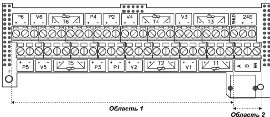
Рисунок Б.3 – Плата подключений вычислителя KAPAT-307-6V6T6P
