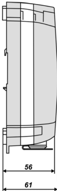
Рисунок А.1 – Габаритные размеры вычислителя KARAT-307
