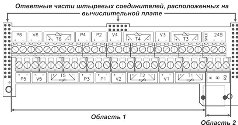
Рисунок Б.3 – Плата подключений вычислителя KARAT-307-6V6T6P
