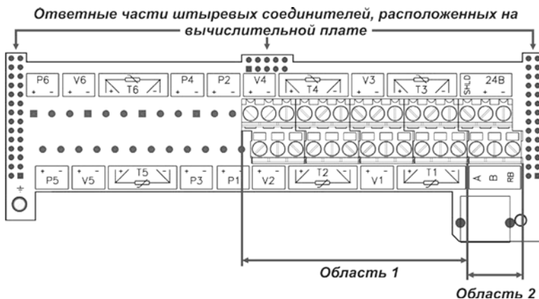
Рисунок Б.1 – Плата подключений вычислителя KARAT-307-4V4T0P
