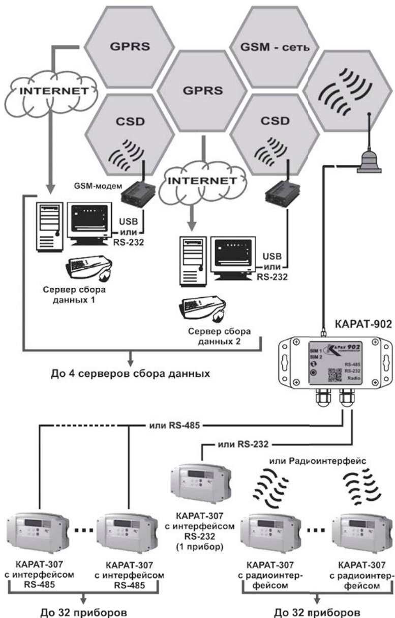
Рисунок В.6 – Принципиальная схема передачи данных с использованием коммуникатора KAPAT-902 по радиоинтерфейсу, контактному интерфейсу и GSM/GPRS сетям
