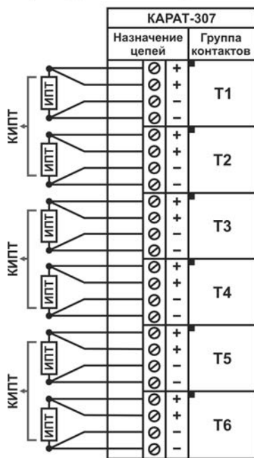
Рисунок 2.6 – Схема подключения КИПТ (ИПТ)
