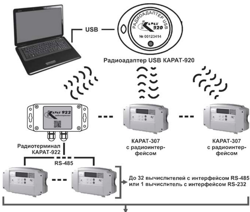
Рисунок В.7 – Принципиальная схема передачи данных по радиоинтерфейсу с использованием радиоадаптера USB KAPAT-920 и радиотерминала KAPAT-922
