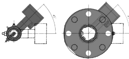
Рисунок 2.3 – Требуемое рабочее положение расходомера
