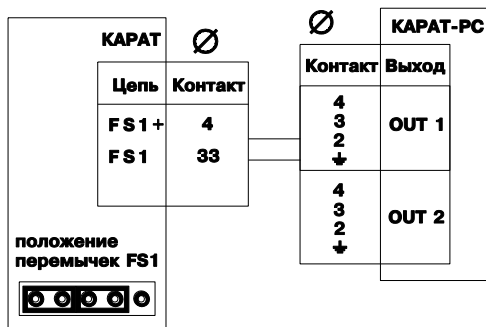
а) Выход типа «открытый коллектор»
