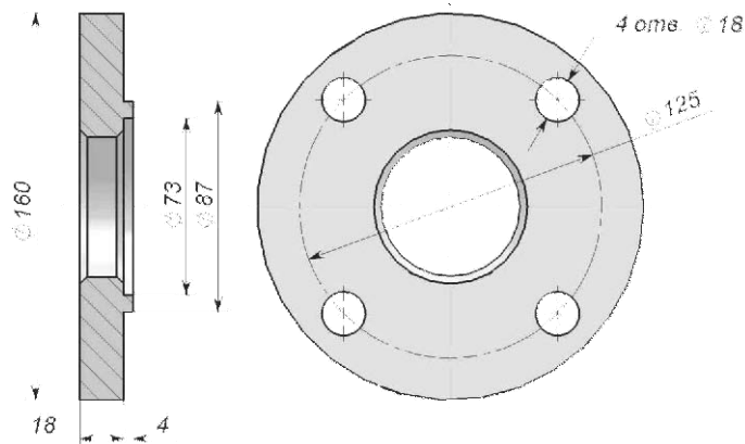
Рисунок Г.3 – Габаритные и установочные размеры КМЧ 2 для КАРАТ-РС-50
