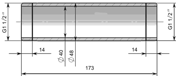
Рисунок Б.2 – Габаритные и установочные размеры монтажной вставки MB-20/32 для расходомера KARAT-PC-20
