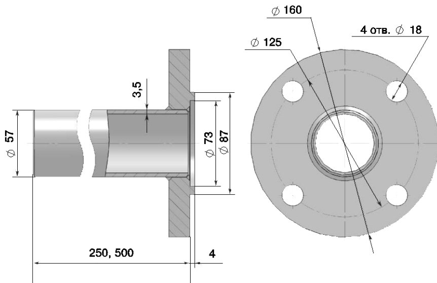
Рисунок Г.4 – Габаритные и установочные размеры КМЧ 3 для КАРАТ-РС-50
