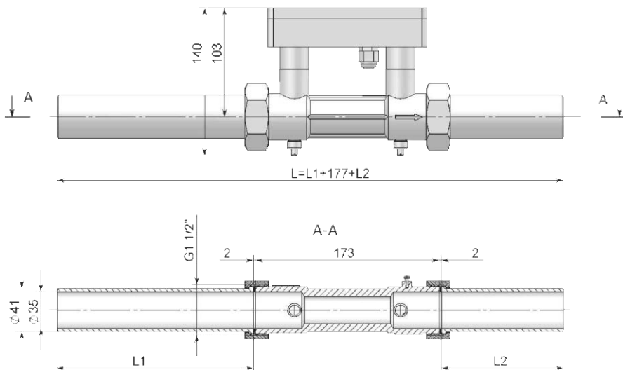
Рисунок В.1 – Габаритные и установочные размеры расходомера KARAT-PC-32
