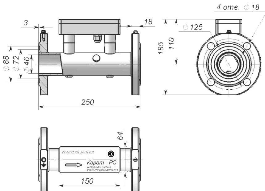
Рисунок Г.1 – Габаритные и установочные размеры расходомера КАРАТ-РС-50
