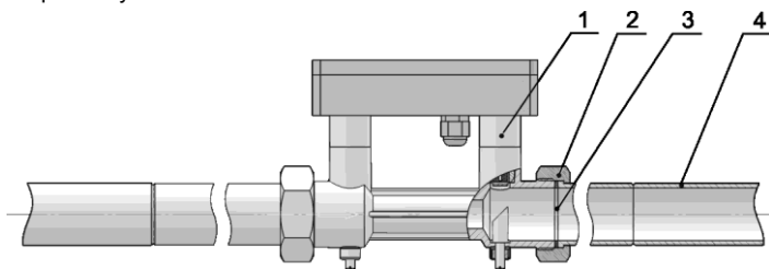
Рисунок А.1 – Схема установки расходомера с резьбовым соединением (Ду 20-32)
