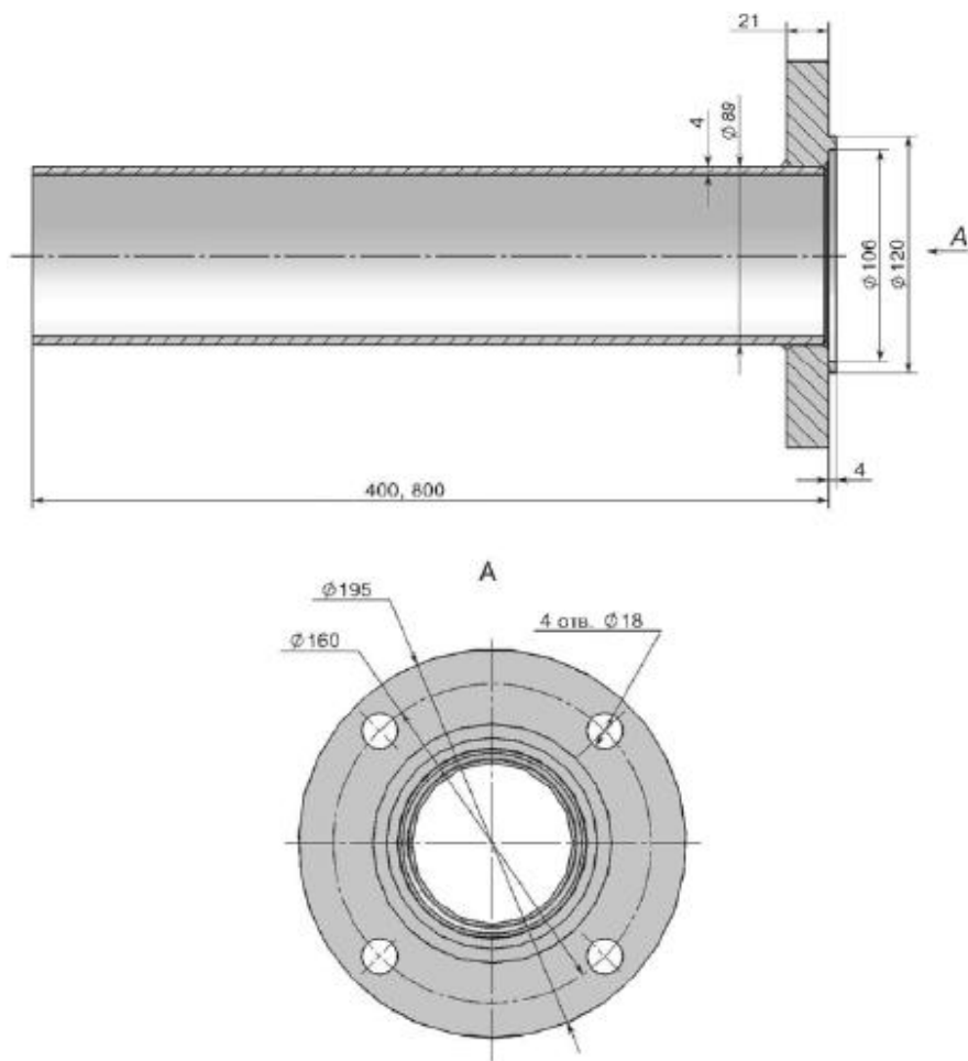
Рисунок Д.4 – Габаритные и установочные размеры КМЧ 3 для КАРАТ-РС-80
