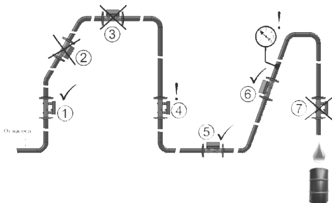
Рисунок 2.2 – Рекомендации по установке и монтажу расходомеров KARAT-PC
