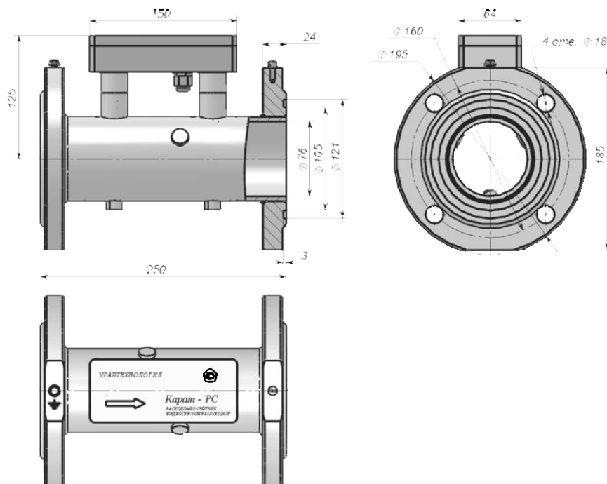
Рисунок Д.1 – Габаритные и установочные размеры расходомера КАРАТ-РС-80
