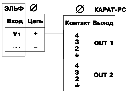
б) Выход типа «гальваническая развязка»
