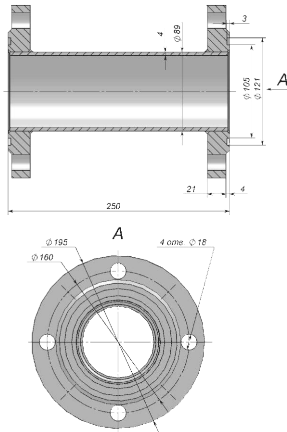
Рисунок Д.2 – Габаритные и установочные размеры монтажной вставки МВ-80 для расходомера КАРАТ-РС-80
