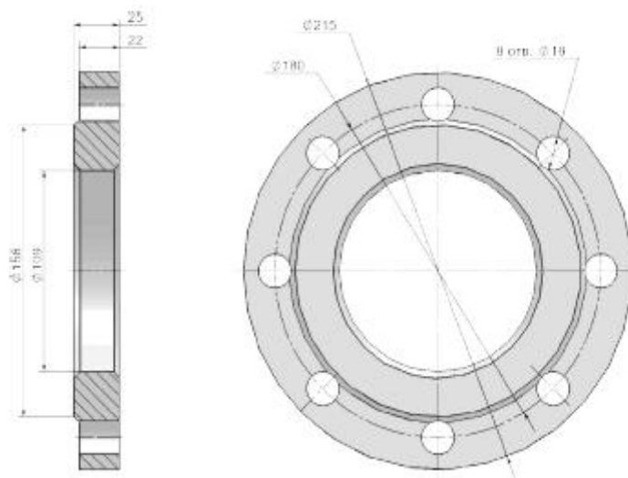
Рисунок Е.2 – Габаритные и установочные размеры монтажной вставки МВ-100 для расходомера КАРАТ-РС-100
