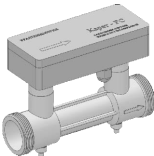
Рисунок 1.2 – Внешний вид ультразвукового расходомера-счетчика жидкости КАРАТ-РС Ду 20, 32 мм
