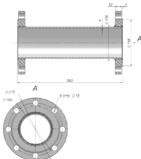
Рисунок Е.2 – Габаритные и установочные размеры монтажной вставки МВ-100 для расходомера КАРАТ-РС-100
