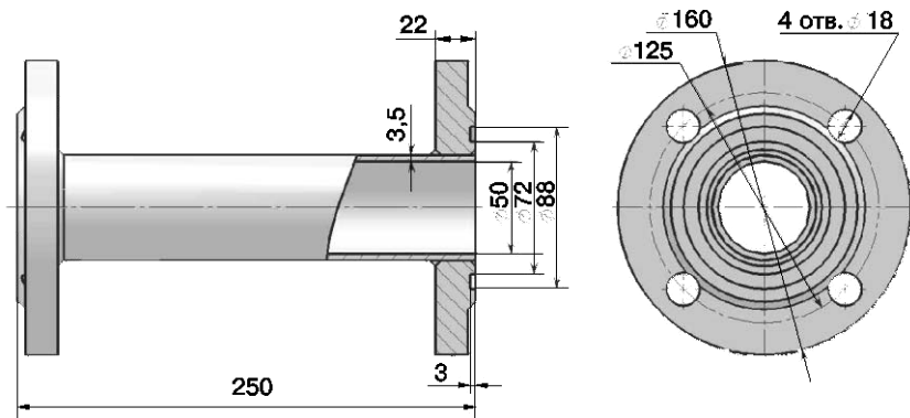
Рисунок Г.2 – Габаритные и установочные размеры монтажной вставки МВ-50 для расходомера КАРАТ-РС-50
