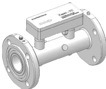
Рисунок 1.3 – Внешний вид ультразвукового расходомера-счетчика жидкости КАРАТ-РС Ду 50, 80 мм
