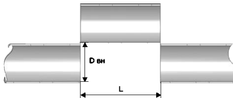
Рисунок 2.5 – Схема вырезки трубопровода для установки расходомера
