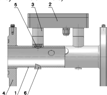
Рисунок 1.5 – Конструкция расходомера KAPAT-PC-50
