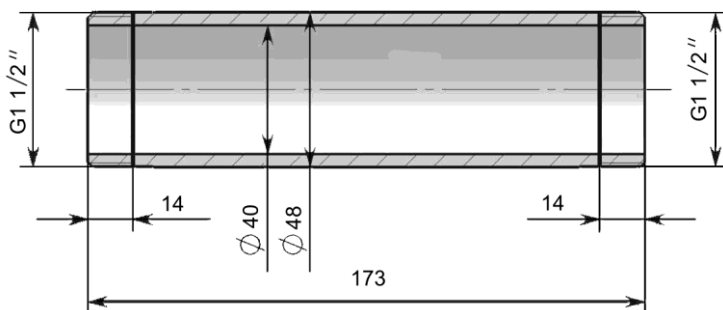
Рисунок В.2 – Габаритные и установочные размеры монтажной вставки MB-20/32 для расходомера KARAT-PC-32
