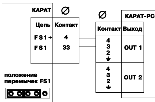
б) Выход типа «гальваническая развязка»
