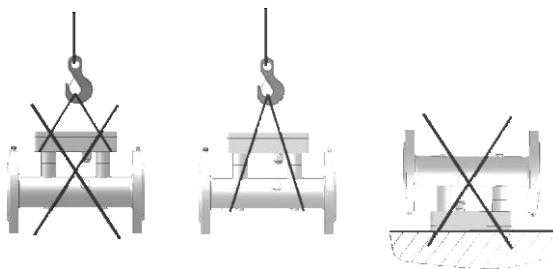
Рисунок 2.4 – Рекомендации по разгрузке и складированию расходомеров
