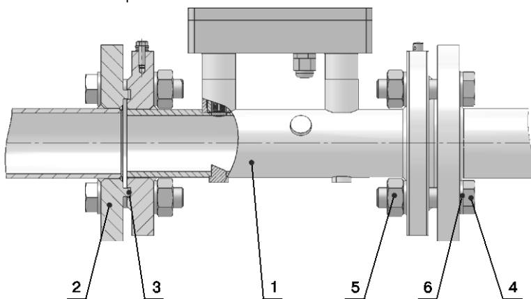
Рисунок А.2 – Схема установки расходомера с фланцевым соединением (Ду 50-100)
