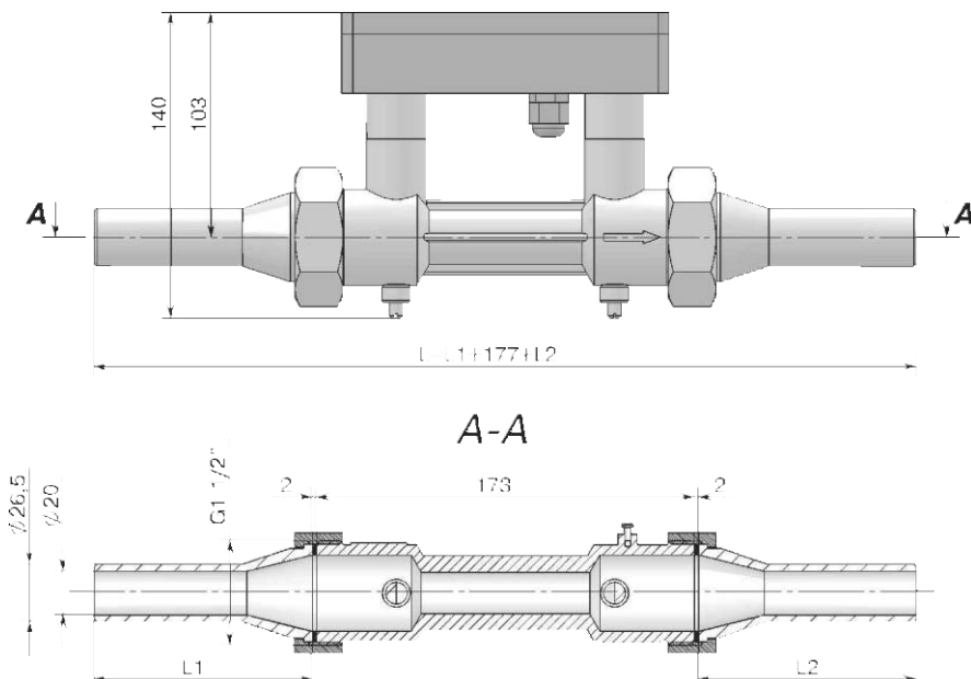
Рисунок Б.1 – Габаритные и установочные размеры расходомера KARAT-PC-20
