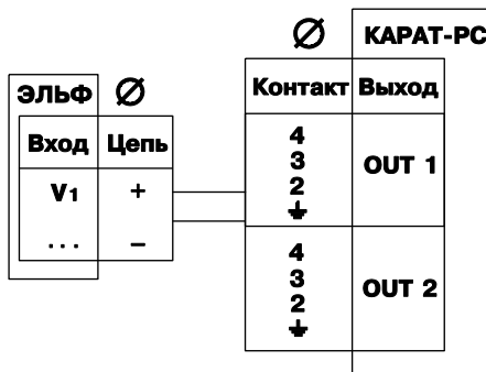
а) Выход типа «открытый коллектор»
