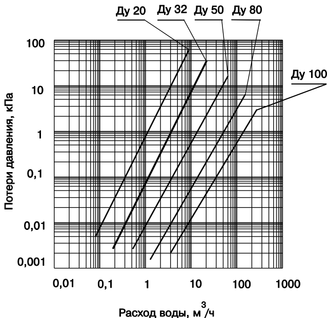
Рисунок 1.1 – Номограмма потери давления расходомера КАРАТ-РС
