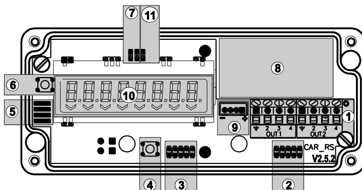
а). Основные элементы расходомера с индикацией в электронном блоке
