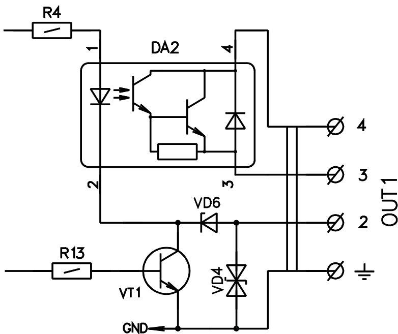
Рисунок Ж.1 – Электрическая схема выходного каскада OUT1 расходомера КАРАТ-РС (схема каскада OUT2 идентична)
