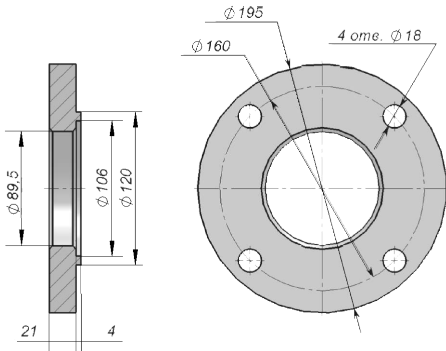
Рисунок Д.3 – Габаритные и установочные размеры КМЧ 2 для КАРАТ-РС-80
