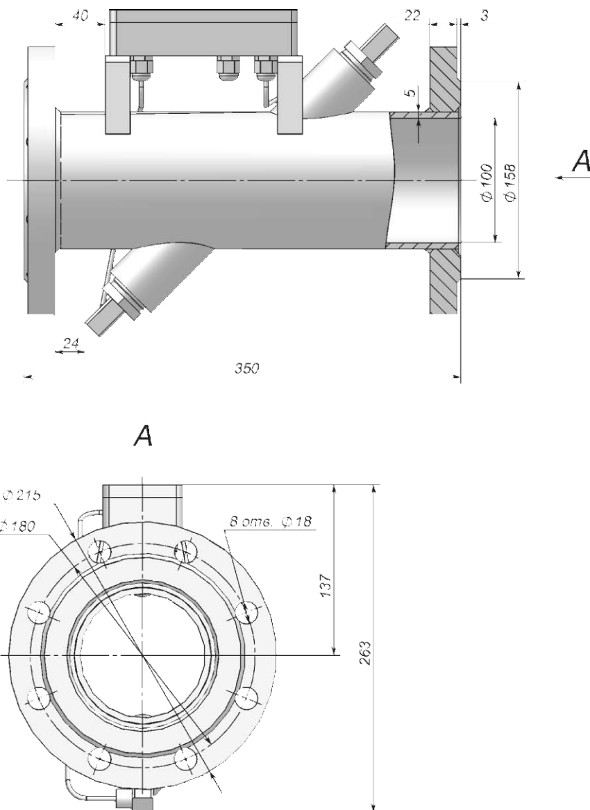
Рисунок Е.1 – Габаритные и установочные размеры расходомера KARAT-PC-100
