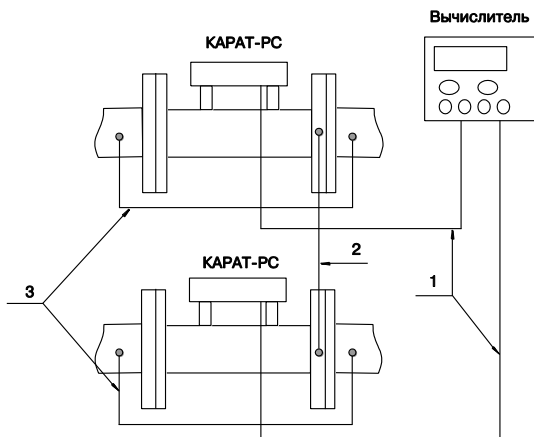
Рисунок 2.7 – Рекомендуемая схема выполнения заземления расходомера КАРАТ-РС
