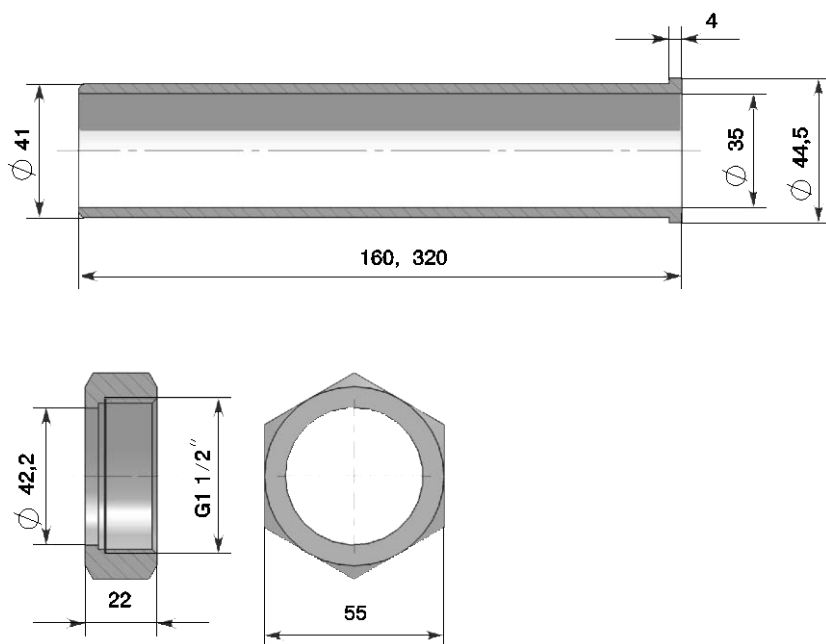
Рисунок В.3 – Габаритные и установочные размеры КМЧ 1 для КАРАТ-РС-32
