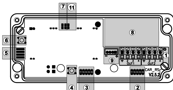
б) Основные элементы расходомера без индикации в электронном блоке
