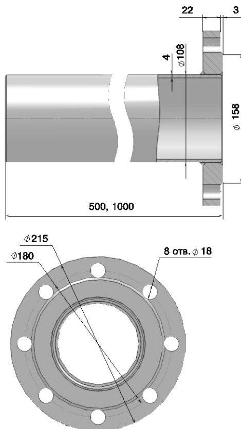
Рисунок Е.4 – Габаритные и установочные размеры КМЧ 3 для КАРАТ-РС-100
