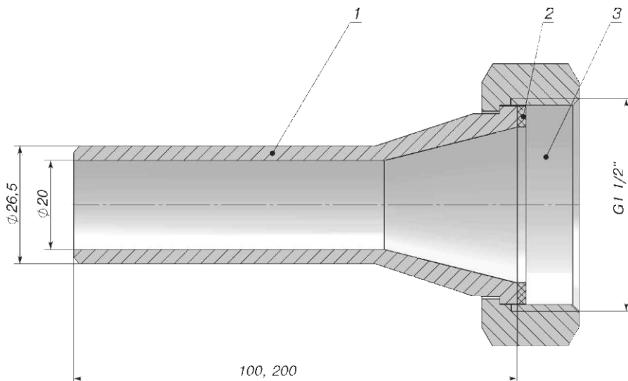
Рисунок Б.3 – Габаритные и установочные размеры КМЧ 1 для KARAT-PC-20
