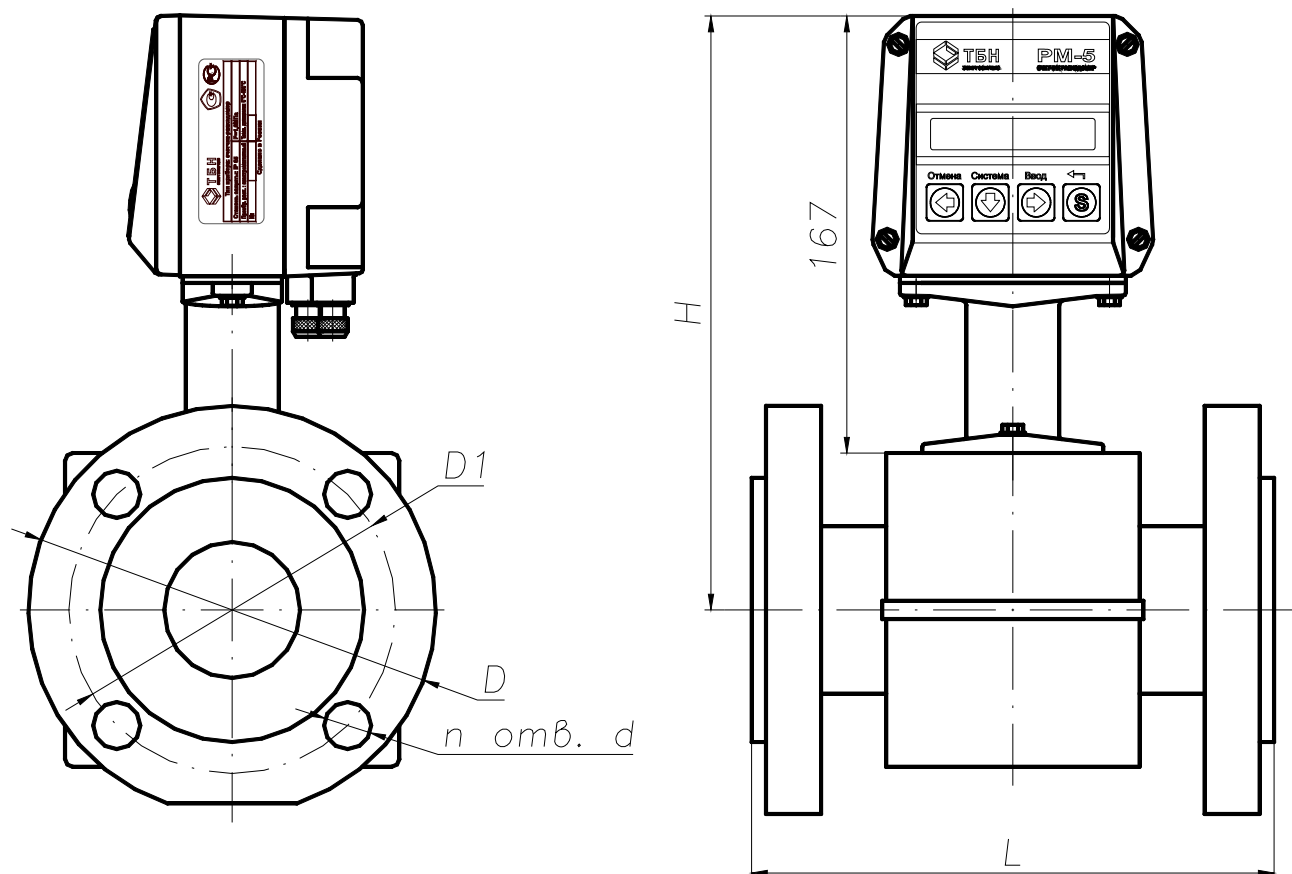
Рисунок В.1 — Фланцевое присоединение датчика расхода Габаритные и присоединительные размеры
