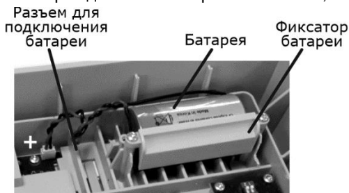
Рис.И.1 – Крепление батареи
