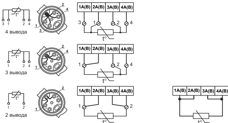
а) Подключение ТС по 4-проводной схеме б) Подключение 2-х проводных ТС
