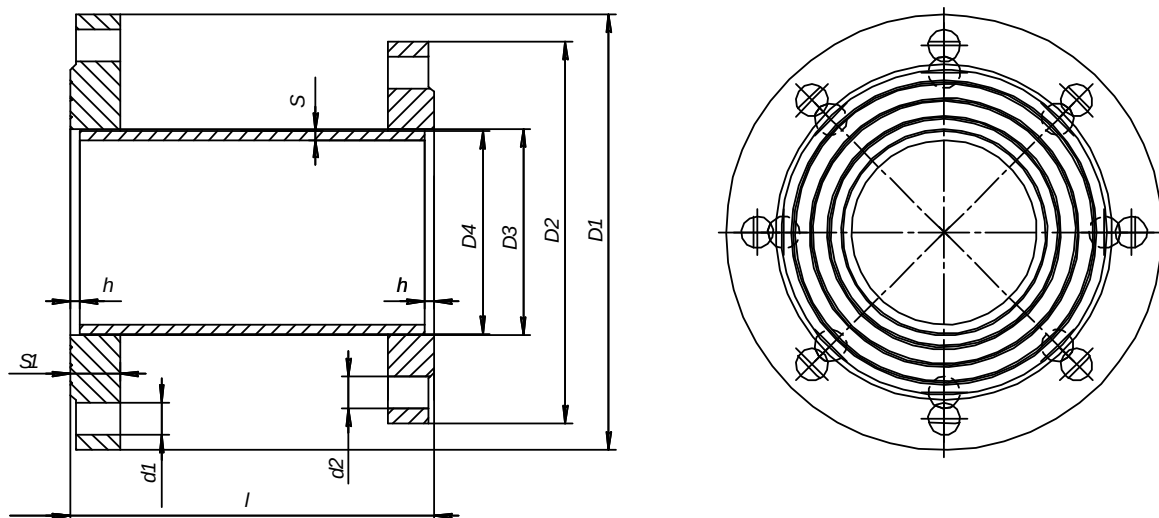
Рис.Л.1. Переходник для монтажа в пластиковый трубопровод.
