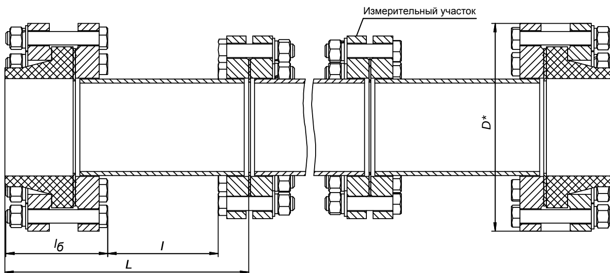
Рис.Л.2. Переходник в сборе.
