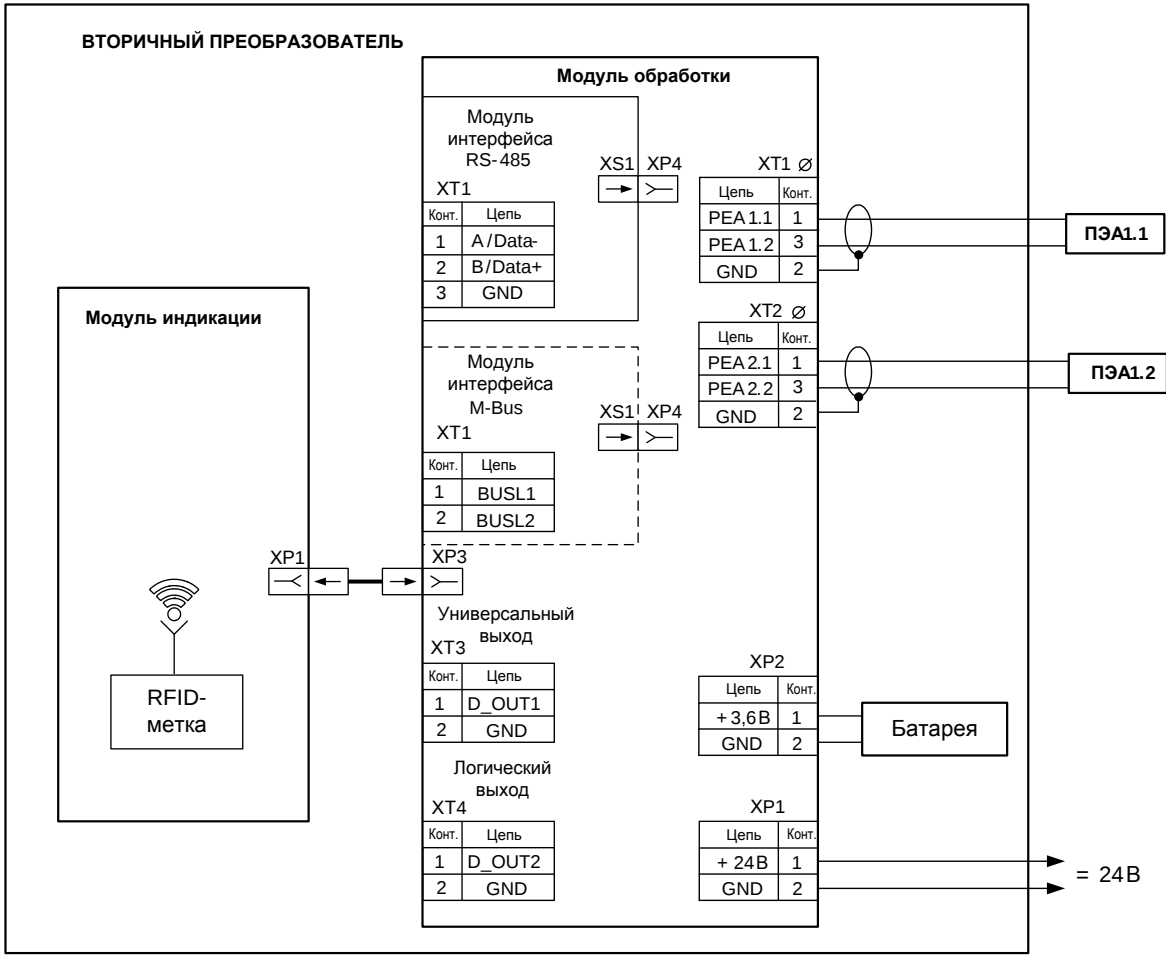
Рис.Б.1. Схема соединений расходомера УРСВ-311 комплектации с RFID-меткой.
