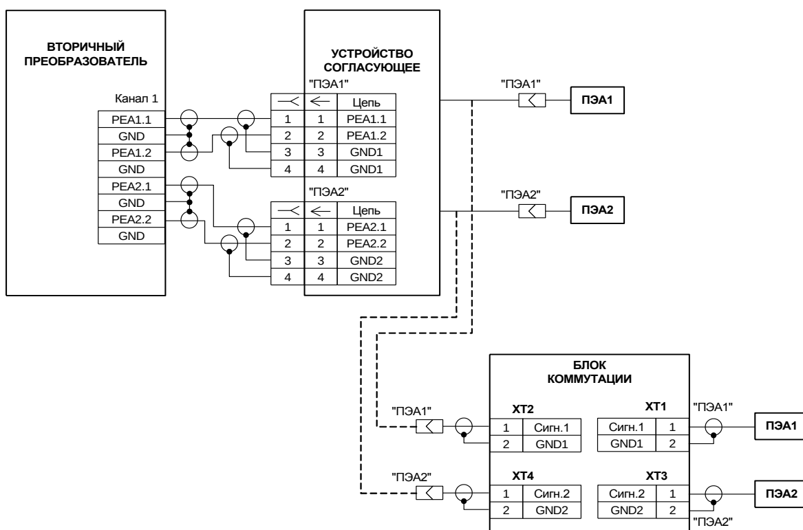
Рис.Г.3. Схема подключения пары ПЭА при симметричной схеме связи.
