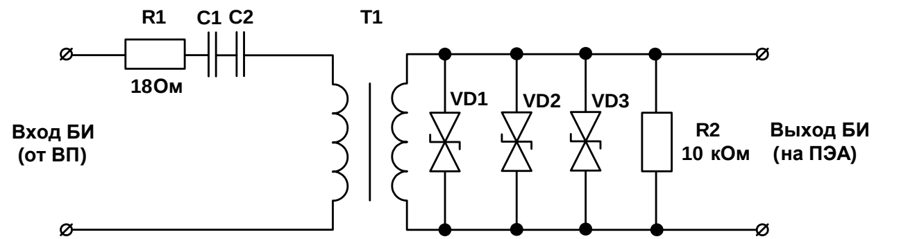
Рис.3. Схема канала искрозащиты
