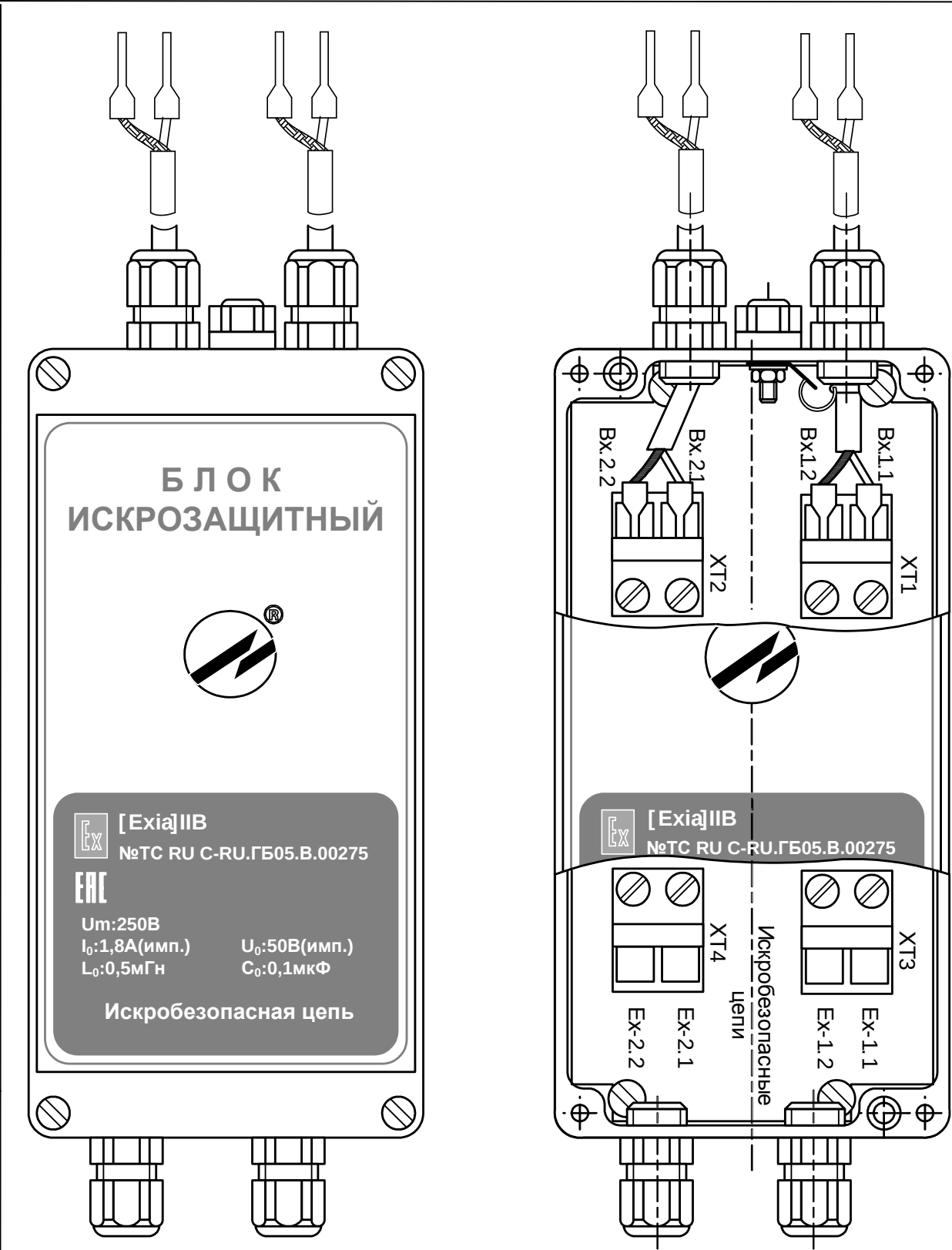
Рис.4. Вид блока искрозащитного
